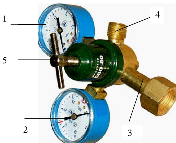
Рис.1 Редуктор БВО-80
