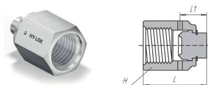
Заглушка с внутренней резьбой
