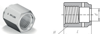
Гайка с внутренней резьбой
