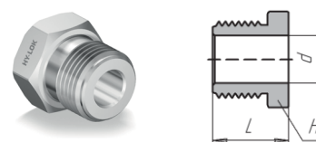
Гайка с наружной резьбой
