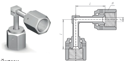
Угольник с гайками
