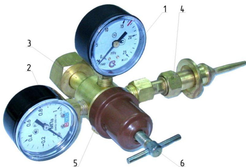
Рис.1 Редуктор БГО-5
