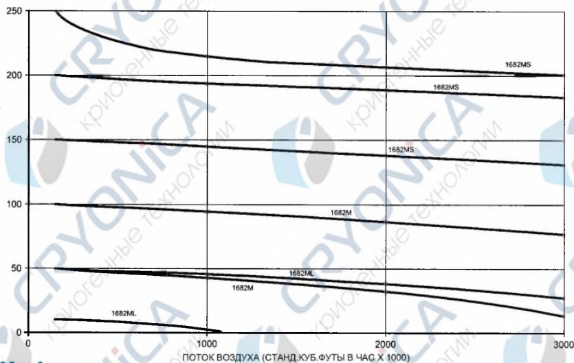
КРИВАЯ ПРОИЗВОДИТЕЛЬНОСТИ РЕГУЛЯТОРОВ СЕРИИ 1682M
